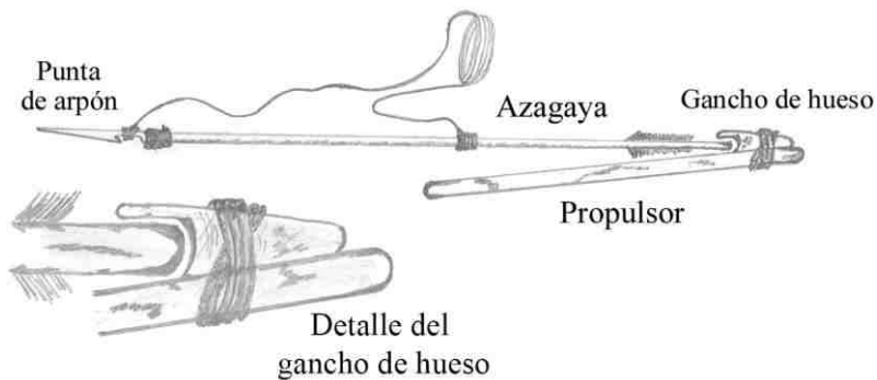
Figura 8. Reconstrucción probable de arma arrojadiza compuesta por propulsor -con el diseño de ganchos encontrados en la Cueva del Negro- y el astil de la azagaya. El gancho de hueso estaría sujeto por medio de ligaduras al extremo distal del propulsor
